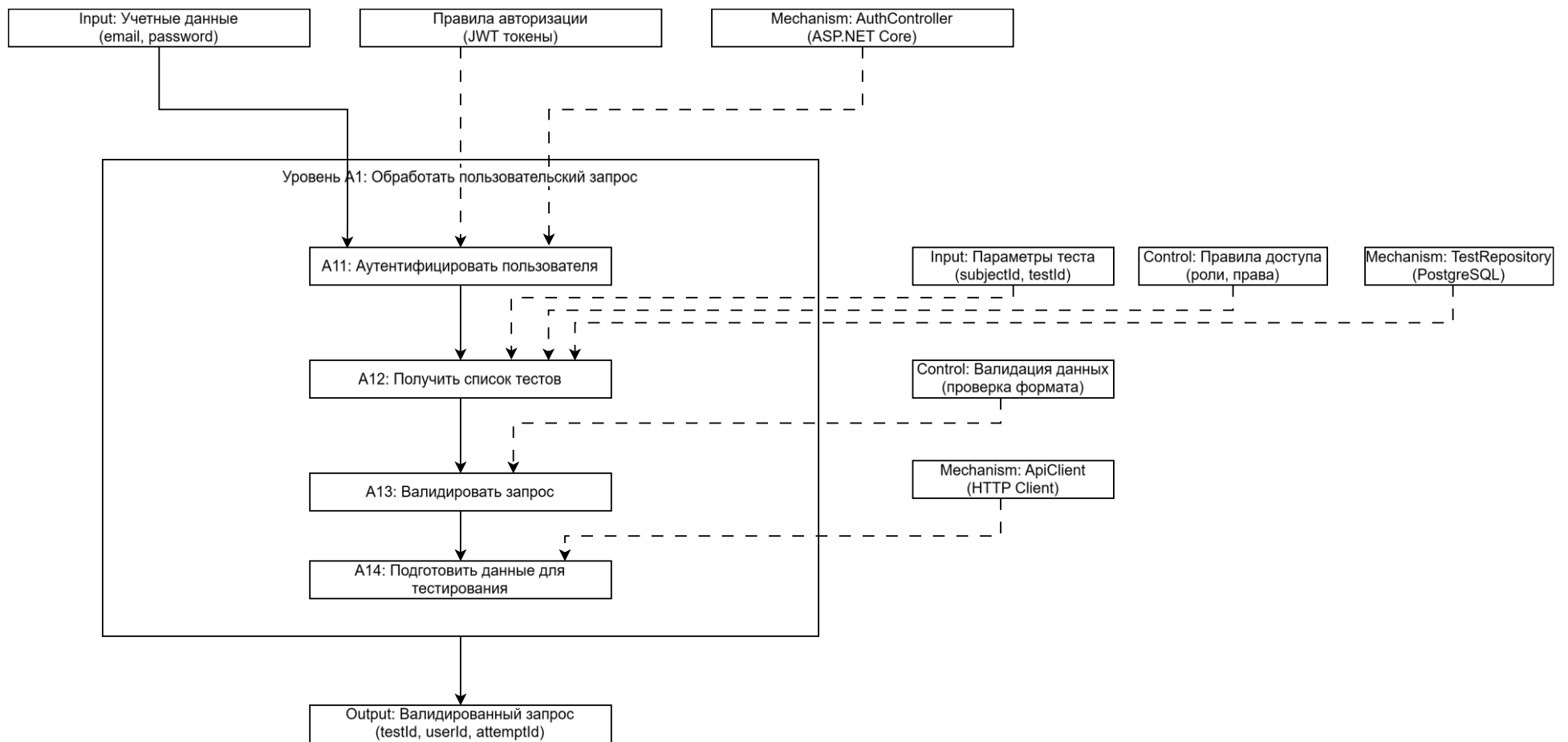
Рисунок 3.9 – Диаграмма IDEF0-A1 «Обработать пользовательский запрос»
