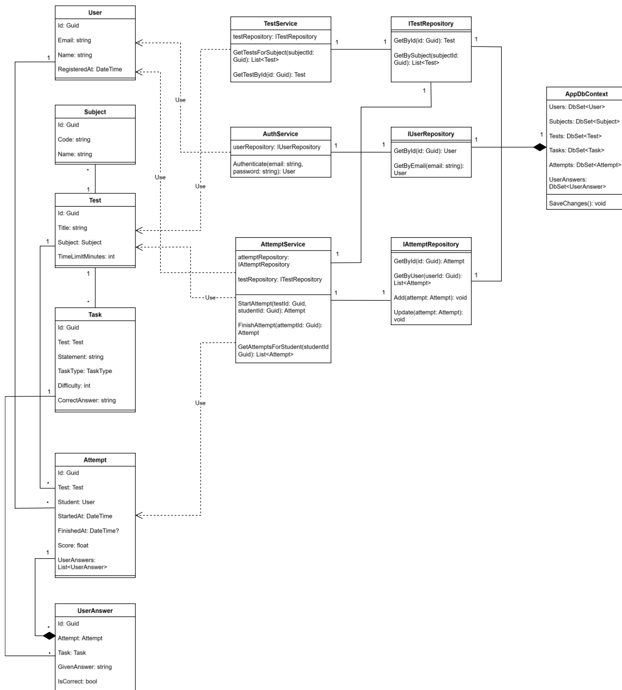
Рисунок 5.1 – Диаграмма классов серверной части (ASP.NET Core)
